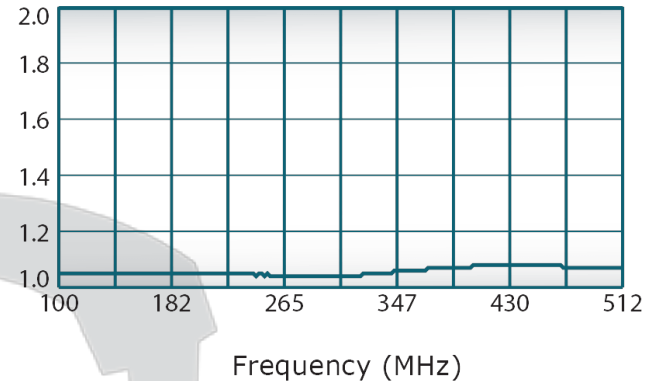
VSWR:
